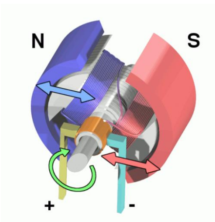
Рис. 11 Приклад використання анімації, що демонструє роботу щіткового електродвигуна постійного струму при вивченні теми уроку: «Загальні відомості про електричні машини»
