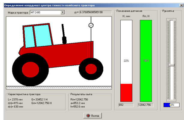
Рис. 4. Визначення координати центру тяжіння трактора
