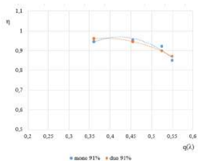
Рис.3 Залежність ККД від газодинамічної функції на вході q(\lambda) при частоті обертання вала 9848,511 об/хв
