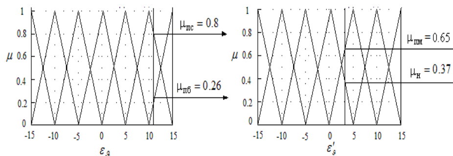
Рис. 4. Процедура вхідного перетворення
