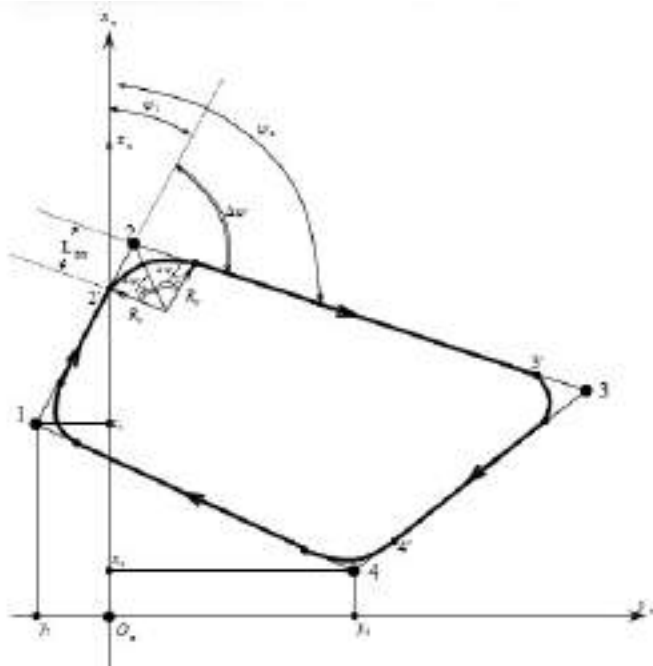
Рис. 2. Маршрут БПЛА на постійній висоті
