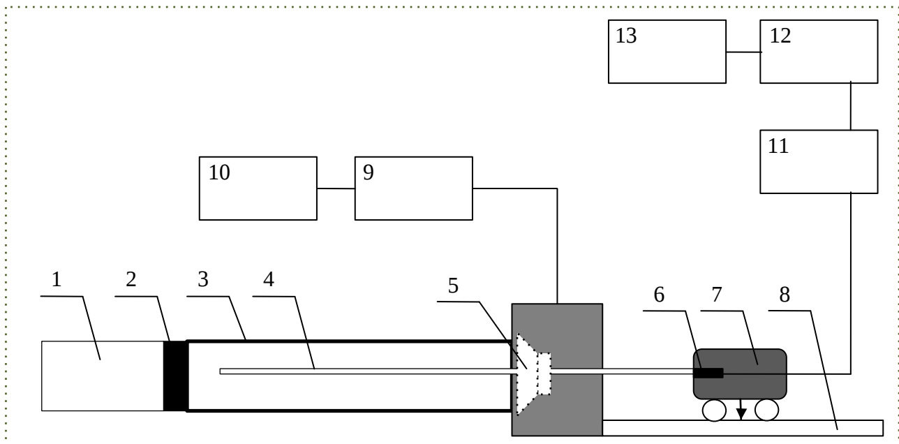
Рис. 3. Схема установки для вимірювання акустичних характеристик ЗПК. 1 – тримач дослідного зразка, 2 – дослідний зразок, 3 – труба інтерферометра (імпедансна труба), 4 – вимірювальна трубка, 5 – звуковий динамік, 6 – мікрофон, 7 – візок, 8 – вимірювальна лінійка, 9 – підсилювач сигналу, 10 – генератор гармонічного сигналу, 11 – вимірювальний підсилювач, 12 – АЦП, 13 – ПК.
