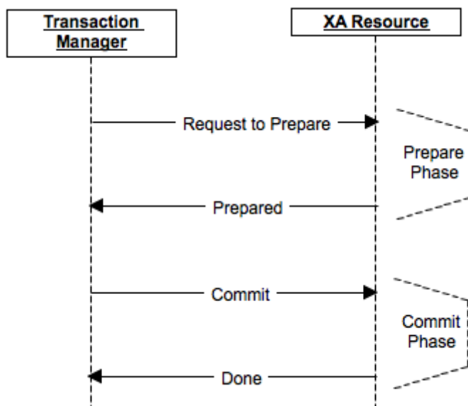
Рис. 1. Ілюстрація роботи шаблону Two-phase-commit
