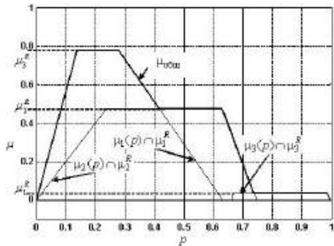
Рис. 5. Процес агрегування функцій належності вихідного сигналу
