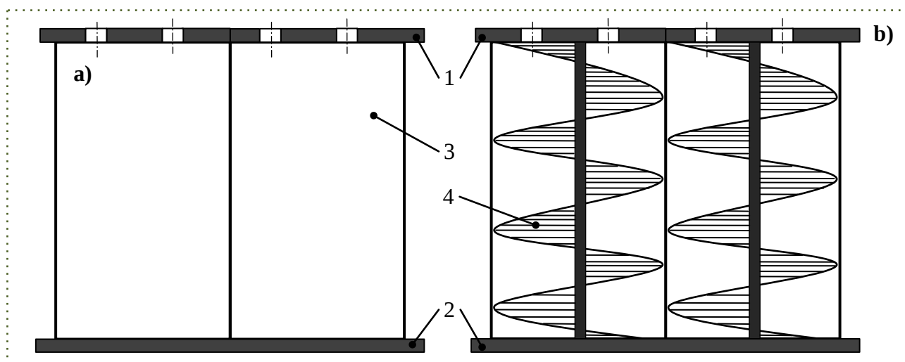
Рис. 2. Порівняння резонансної конструкції ЗПК a) та модифікованої конструкції ЗПК b) . 1 – перфорована обшивка, 2 – суцільна обшивка, 3 – наповнювач ЗПК, 4 – модифікований наповнювач ЗПК.
