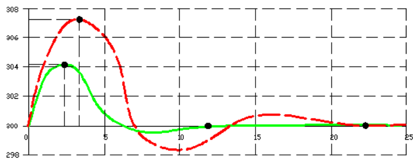
Рис. 6. Перехідні процеси стабілізації висоти БПЛА з використанням ПД- регулятора та ІСК в умовах пориву вітру з постійною швидкістю 15 м/с,
