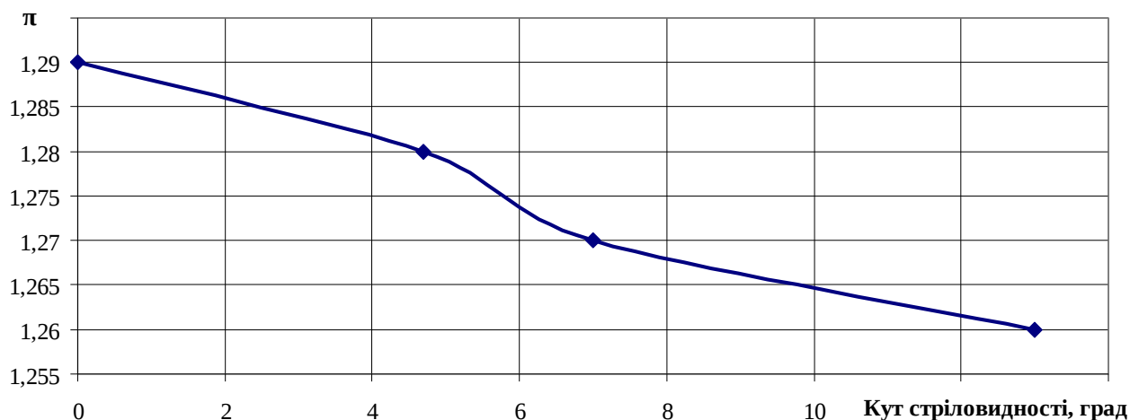
Рис. 1. Залежність кута стріловидності передньої кромки лопаток вентилятора від ступеня підвищення тиску у вентиляторі \pi
