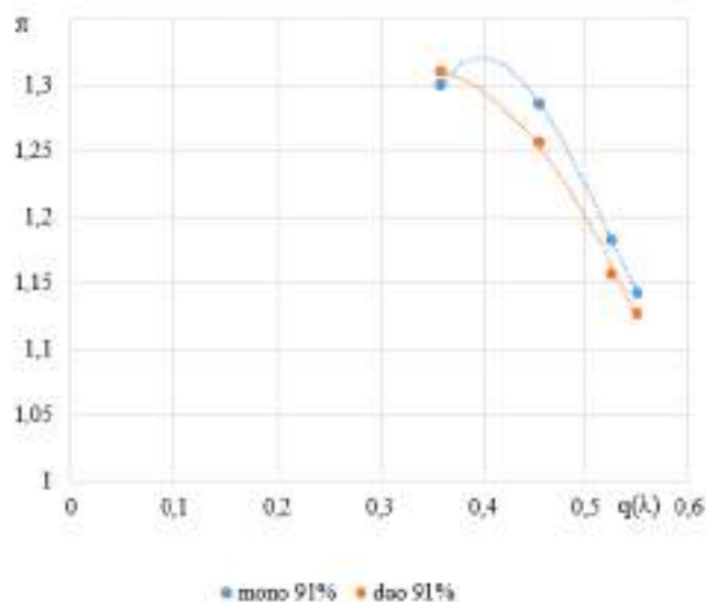
Рис.2 Залежність ступеня підвищення тиску від газодинамічної функції на вході q(\lambda) при частоті обертання вала 9848,511 об/хв
