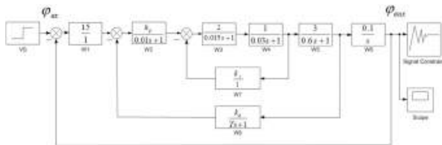
Рис. 2. Імітаційна модель САК приводом робота-маніпулятора
