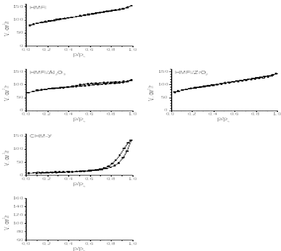
Рис. 2. Ізотерми адсорбції/десорбції азоту вихідного НМФІ та модифікованих НМФІ/ \text{Al}_2\text{O}_3 , НМФІ/ \text{ZrO}_2 цеолітних каталізаторів, а також металоксидного каталізатора СНМ-У.
